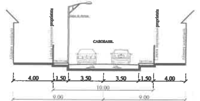
PROFIL TRANSVERSAL 2-2 SCARA 1:200
