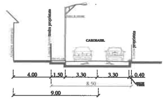
PROFIL TRANSVERSAL 3-3 SCARA 1:200
