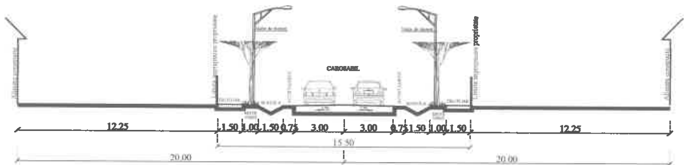
PROFIL TRANSVERSAL 1-1 SCARA 1:200
